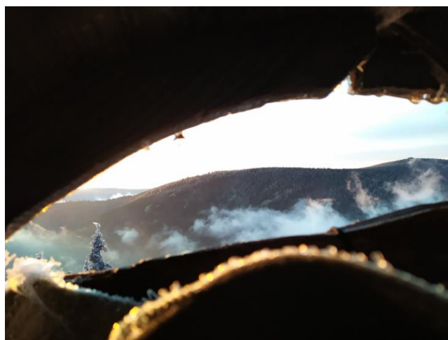
3 er premio 2021: "Vista de la intersección de una elipse y una parábola " de Martin Zdeněk, Gymnázium Čajkovského de Olomouc
